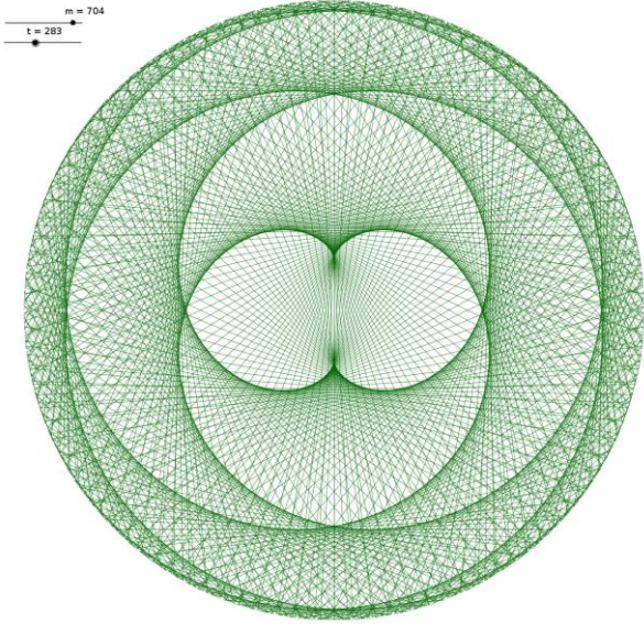
m = 704 ; t = 283
