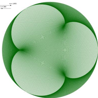
m = 1455 ; t = 364
