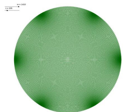
m = 1410 ; t = 235
