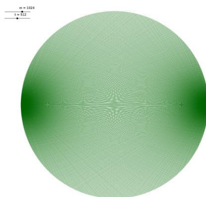
m = 1024 ; t = 512
